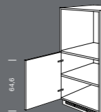
SUB Colonna per forno Mueble columna para horno Altezza nicchia Distancia mueble alto/ bajo 58,5–59,5 cm, Larghezza Ancho 60 cm
