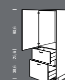
SUA Colonna Mueble columna Altezza nicchia Distancia mueble alto/ bajo 88 cm, Larghezza Ancho 60 cm
