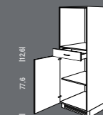
SUBS Colonna per forno Mueble columna para horno Altezza nicchia Altura del hueco 58,5 – 59,5 cm, Larghezza Ancho 60 cm
