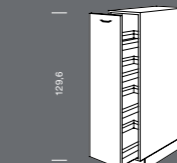
SA Colonna per provviste Mueble columna despensero Larghezza Ancho 30, 45 cm
